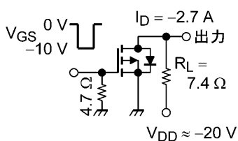
図 6.2.1 スwitching時間の測定回路例 (P-ch) 図 6.2.2 スwitching時間の測定回路例 (N-ch)
