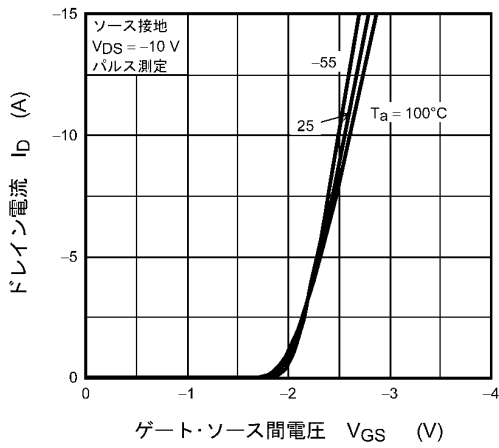
図 8.1.3 ID - VGS
