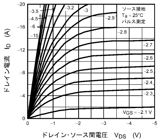
図 8.1.2 ID - VDS
